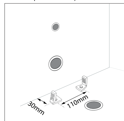
Esquema de fixação ao solo
